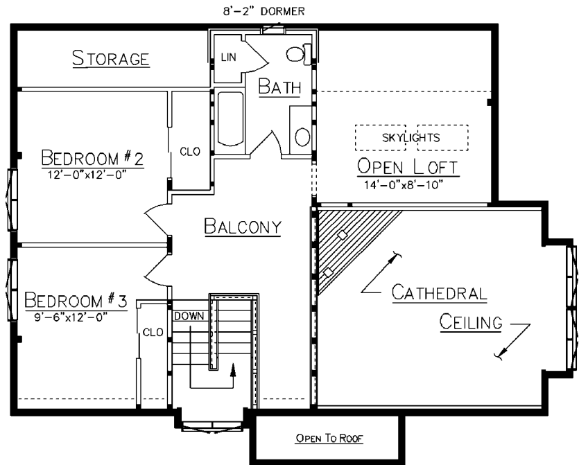
LOFT PLAN
