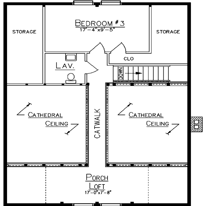
LOFT PLAN
