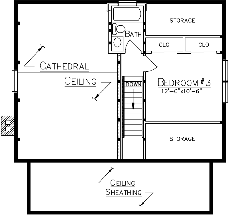
LOFT PLAN
