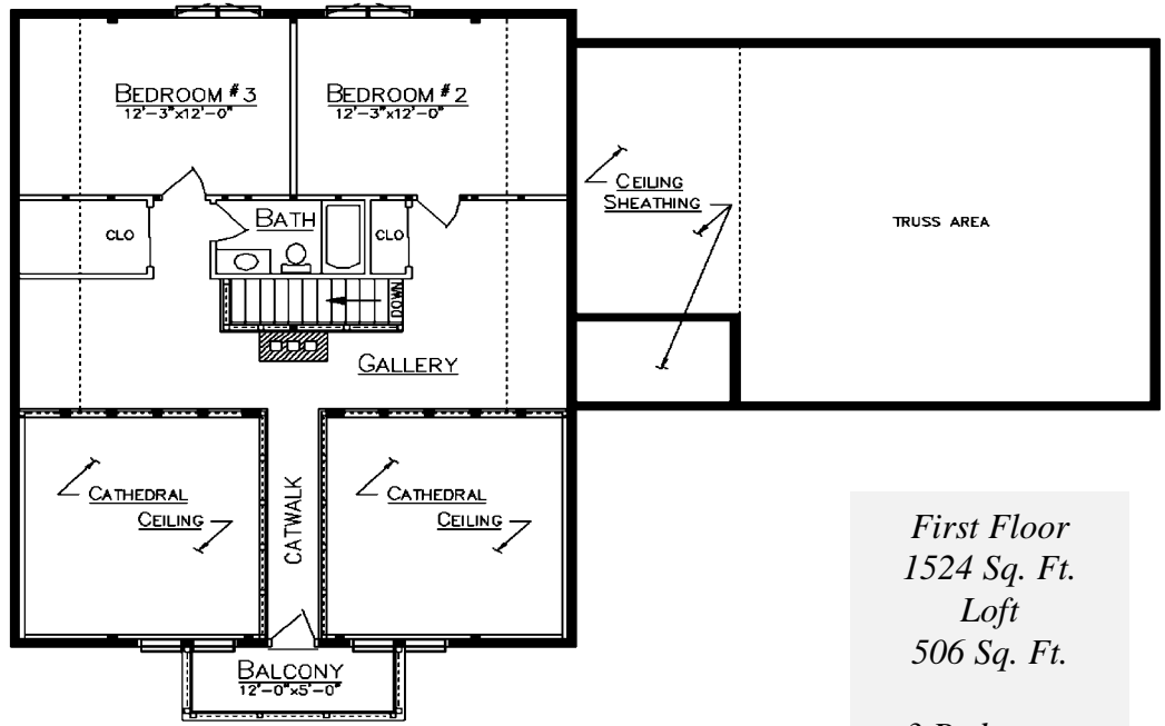
LOFT PLAN
