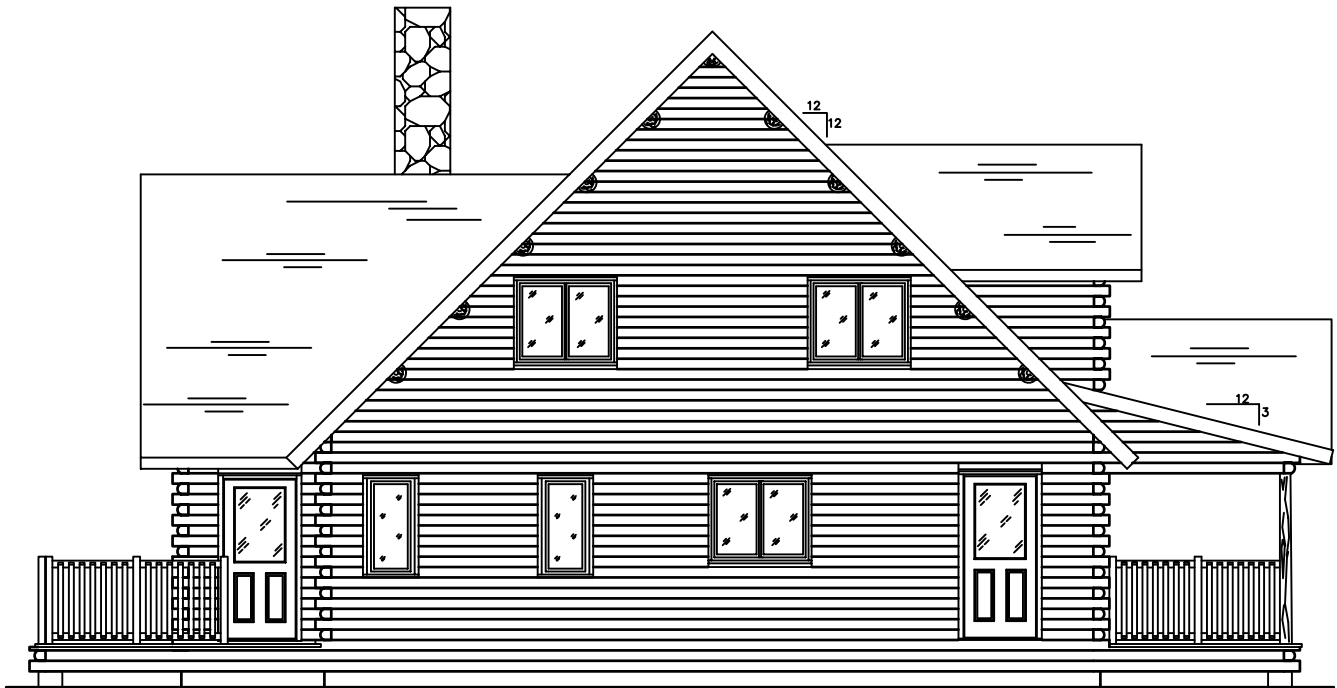
ELEVATION 'D'
