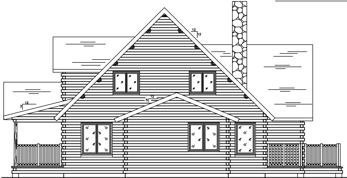
ELEVATION 'B'
