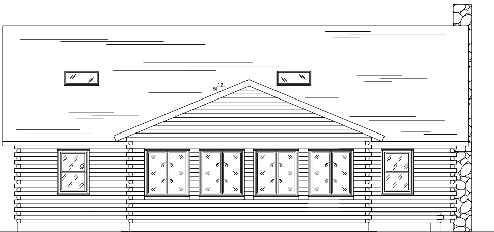
ELEVATION 'C'
