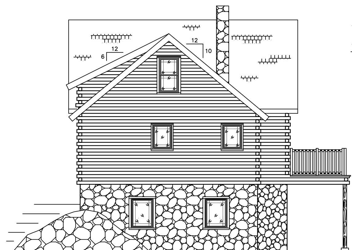
ELEVATION 'D'
