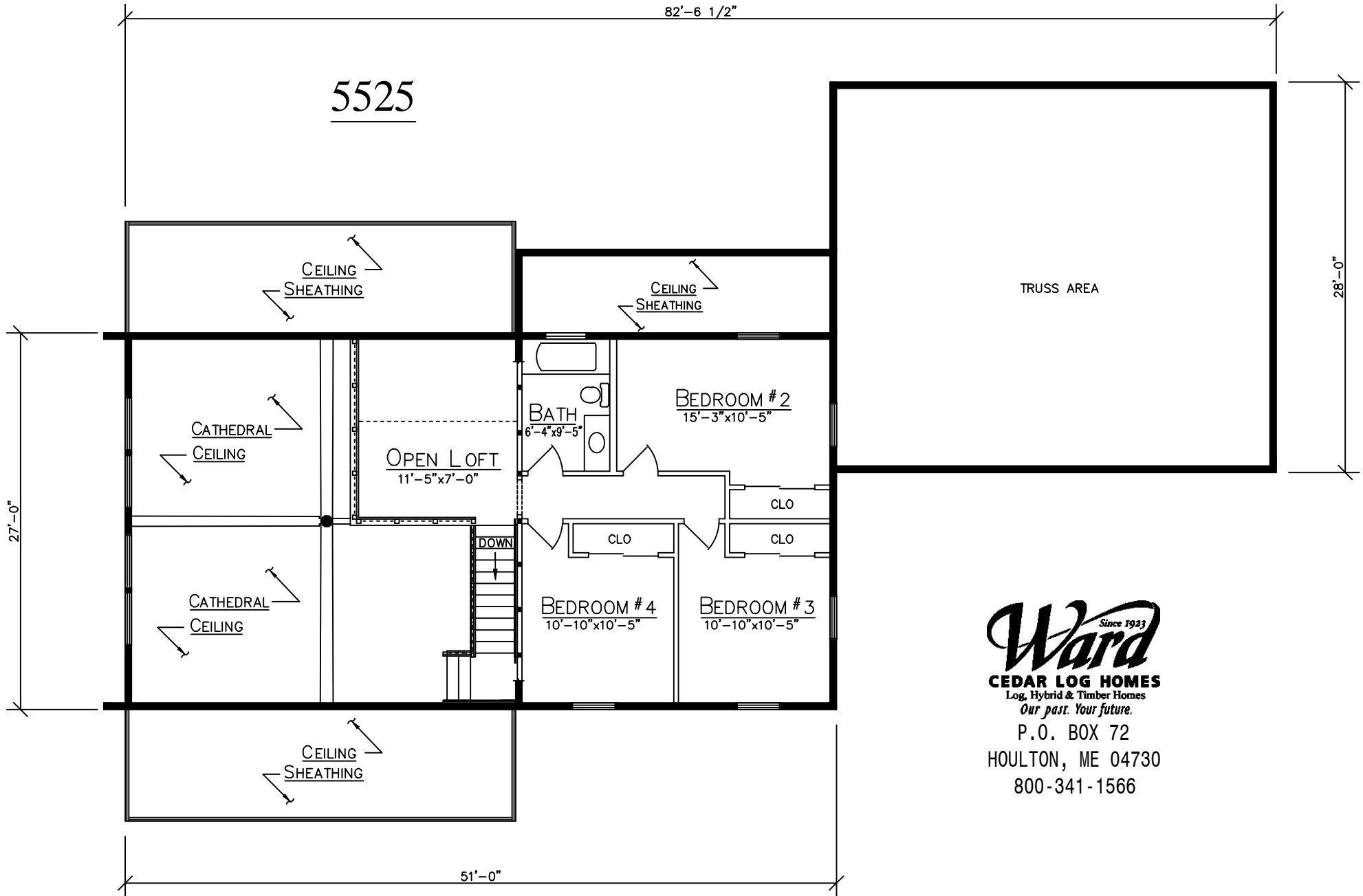
LOFT PLAN
