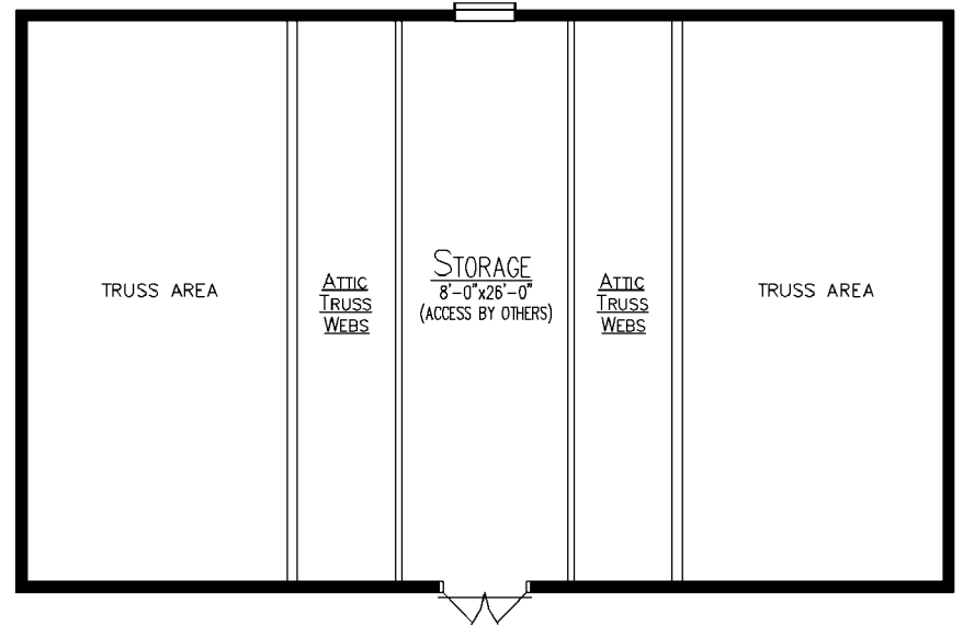
LOFT PLAN
