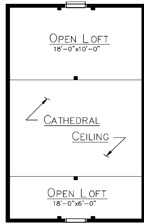
LOFT PLAN
