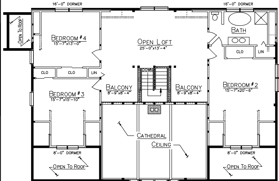
LOFT PLAN
