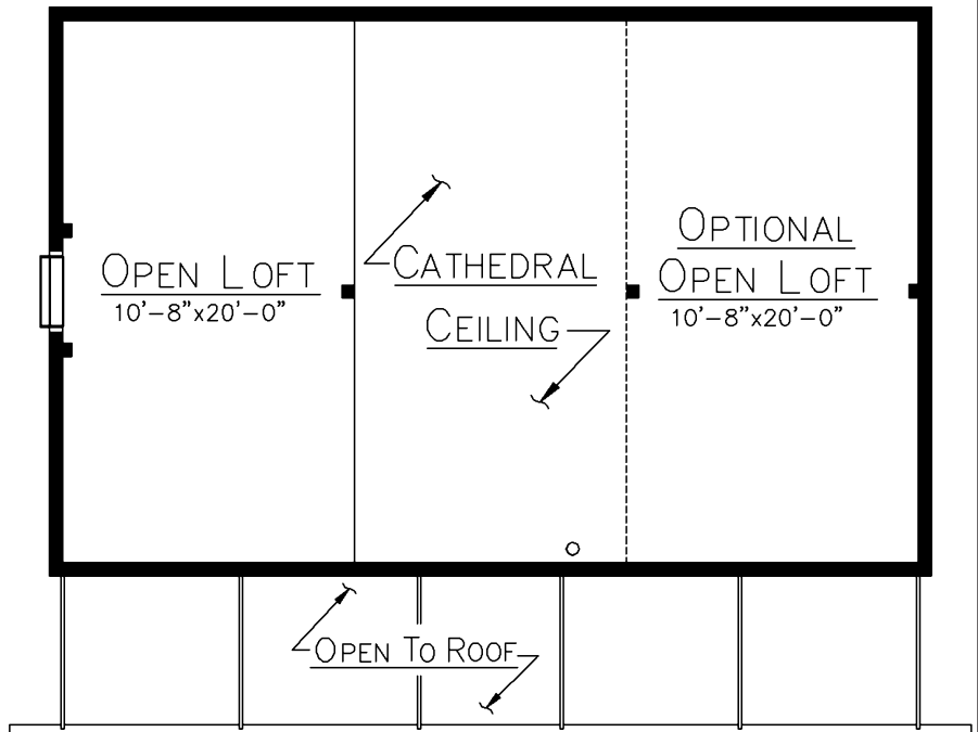
LOFT PLAN
