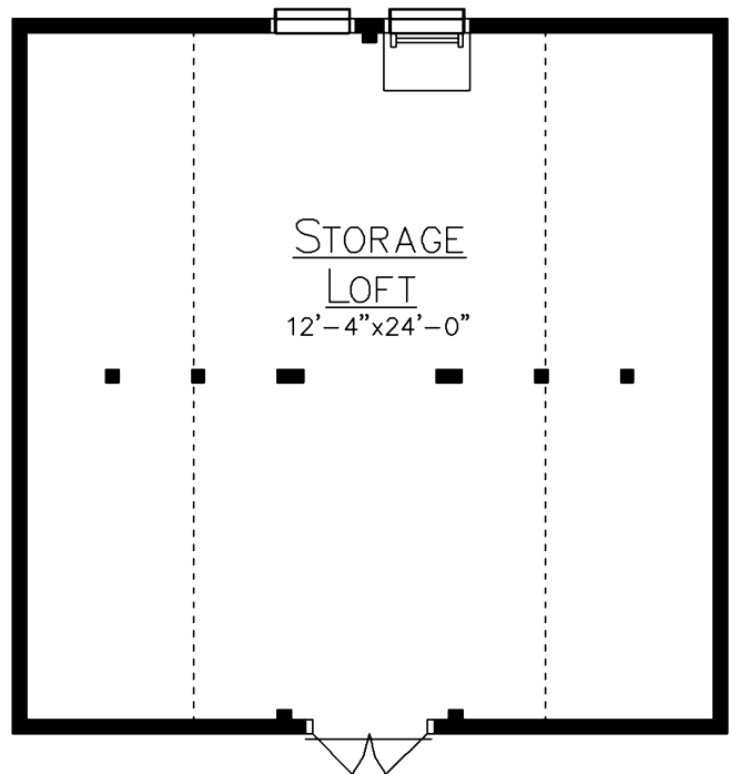
LOFT PLAN
