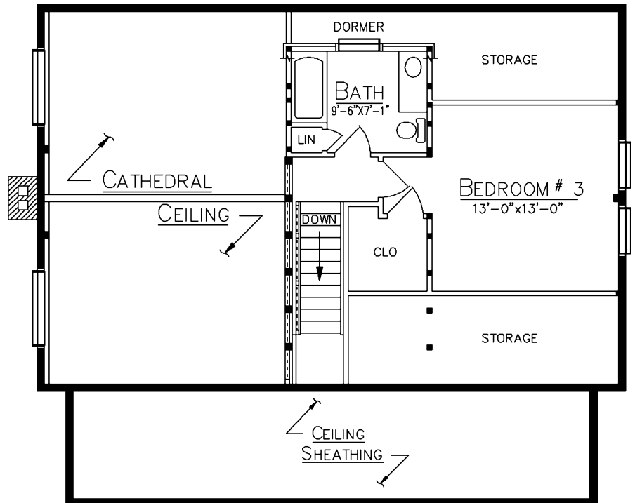
LOFT PLAN
