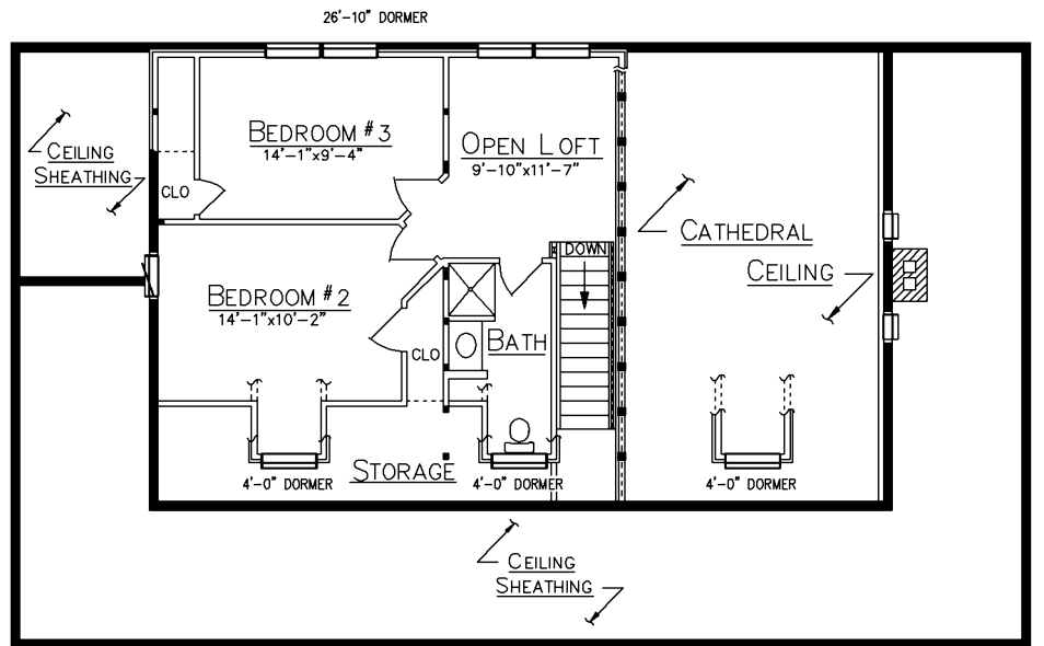
LOFT PLAN
